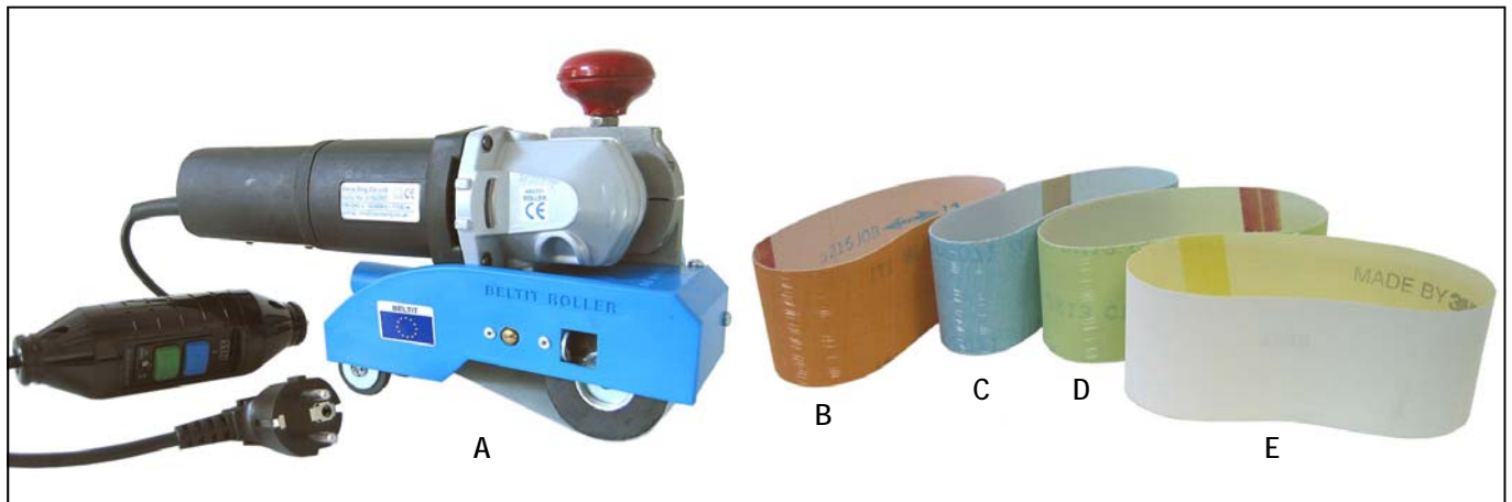
A: 3M Trizact/ Beltit roller.
